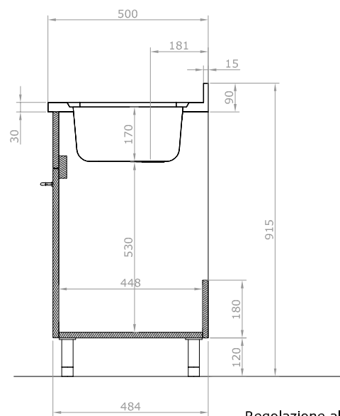
SEZ. A-A
